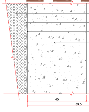
TIPO 14: MUROS BLOQUE
