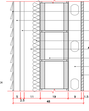
TIPO 11: FACHADA CON BLOQUE
