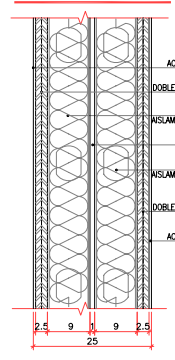
TIPO 3: AULA <--> AULA 57DBA
