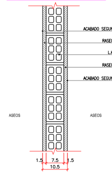
TIPO 7: TABIQUES INTERIORES ASEOS
