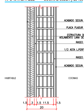
TIPO 1: HABITABLE <--> COCINAS 50DBA y EI-180
