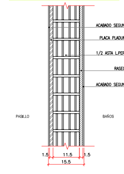
TIPO 6: PASILLO <--> BAÑOS 45DBA y EI-120
