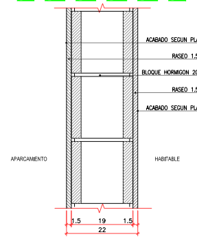
TIPO 8: APARCAMIENTO <--> HABITABLE 45DBA
