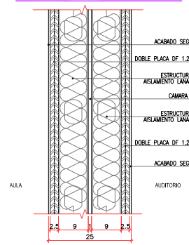
TIPO 4: AULA <-> AUDITORIO 57DBA y EI-120
