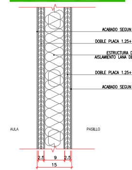
TIPO 5: AULA <-> PASILLO 51DBA
