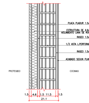
TIPO 2: PROTEGIDO <-> COCINAS 56DBA y EI-180
