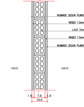
TIPO 7: TABIQUES INTERIORES ASEOS
