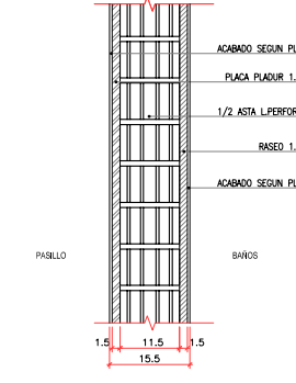
TIPO 6: PASILLO <--> BAÑOS 45DBA y EI>120
