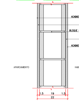
TIPO 8: APARCAMIENTO <--> HABITABLE 45DBA
