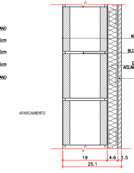
TIPO 9: APARCAMIENTO <--> PROTEGIDO 55DBA
