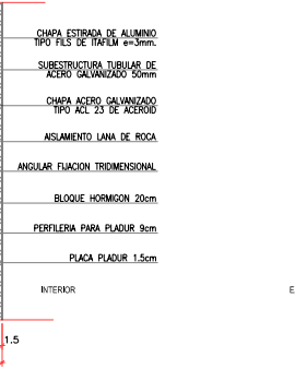
TIPO 12: FACHADA CON MURO
