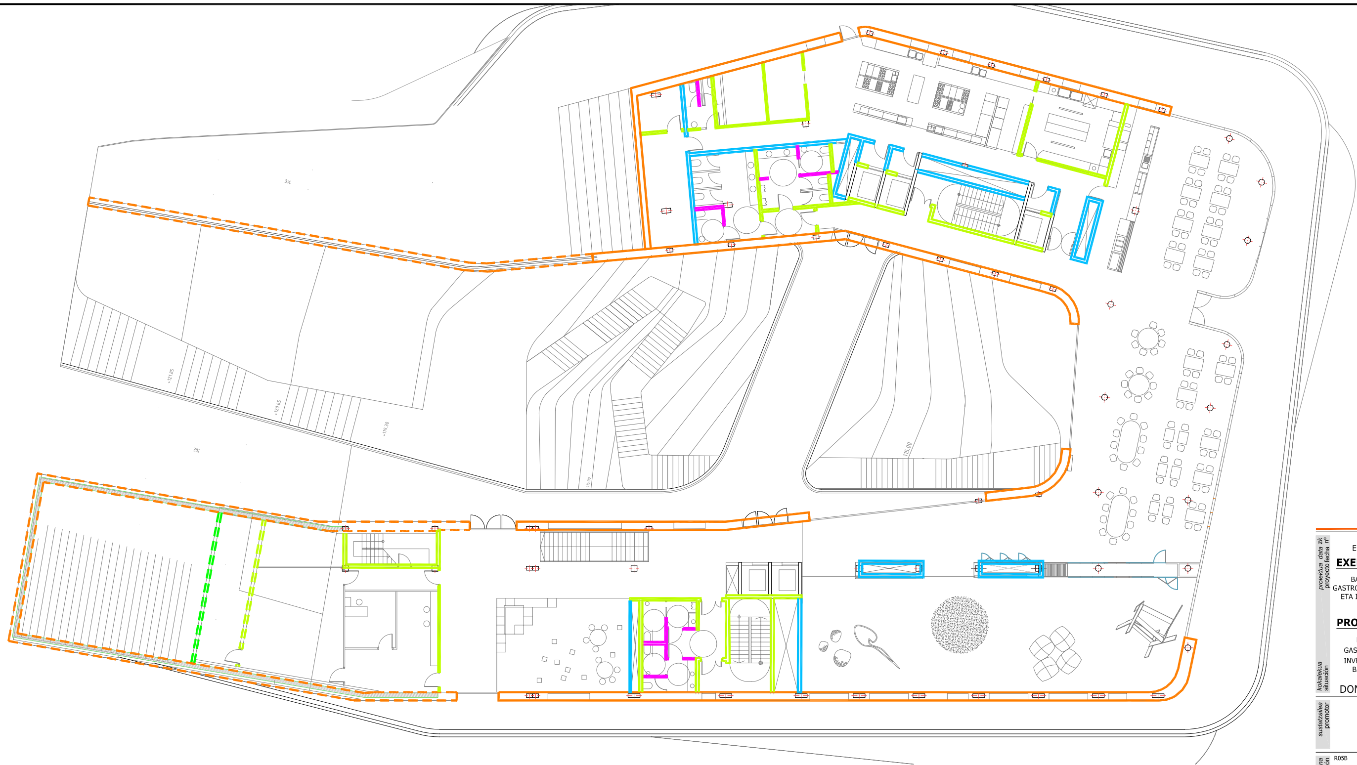
TIPO 1: HABITABLE <--> COCINAS 50DBA y EI>180
