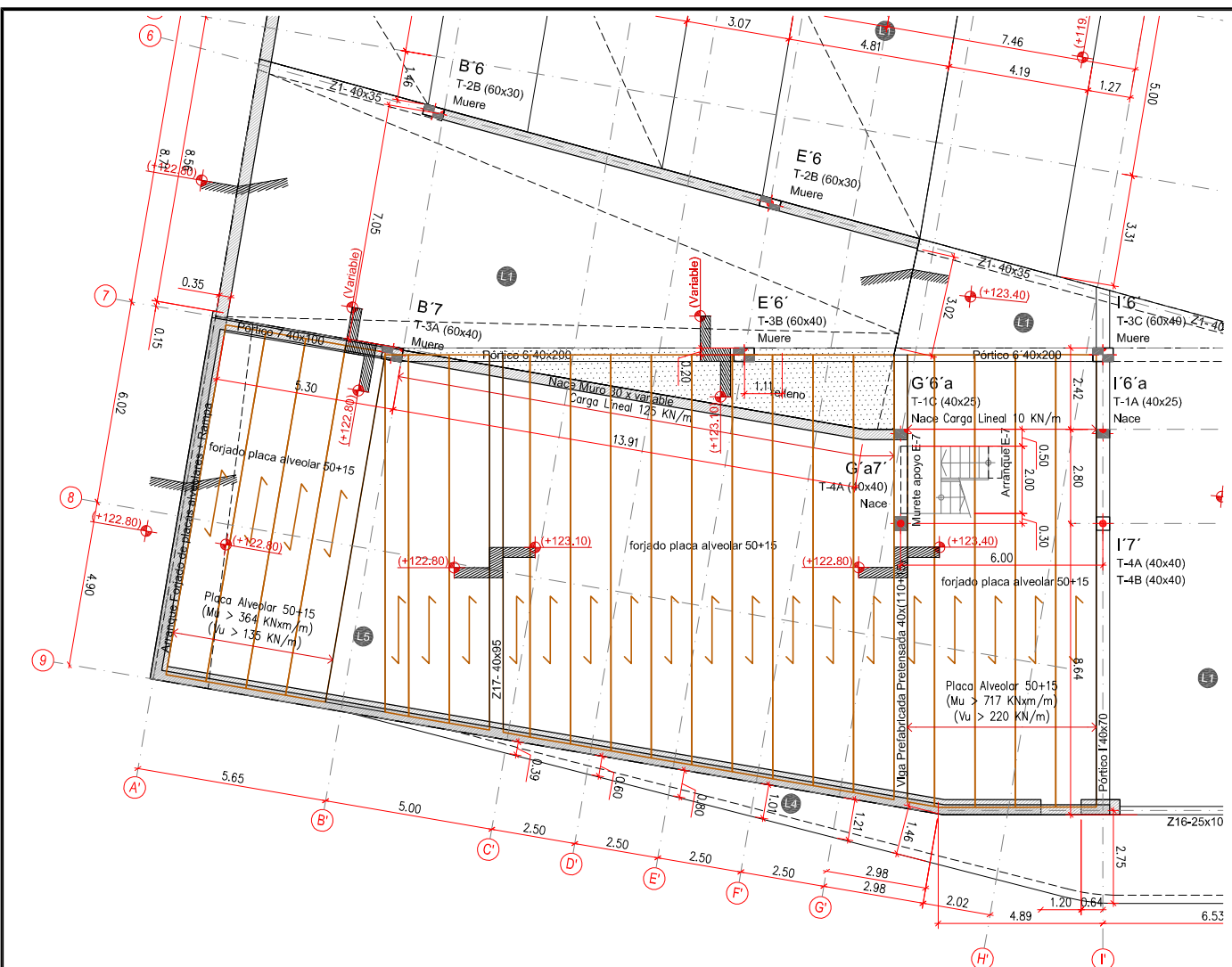
FORJADOS DE PLACA PREFABRICADA PLANTA P0 COTA +119.15 Escala A1:1/100 - A3:1/200
