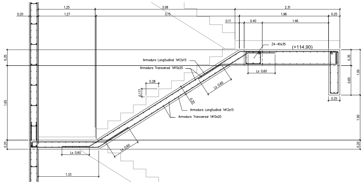
ESCALERA E1. DETALLE B3 Escala A1:1/25 - A3:1/50
