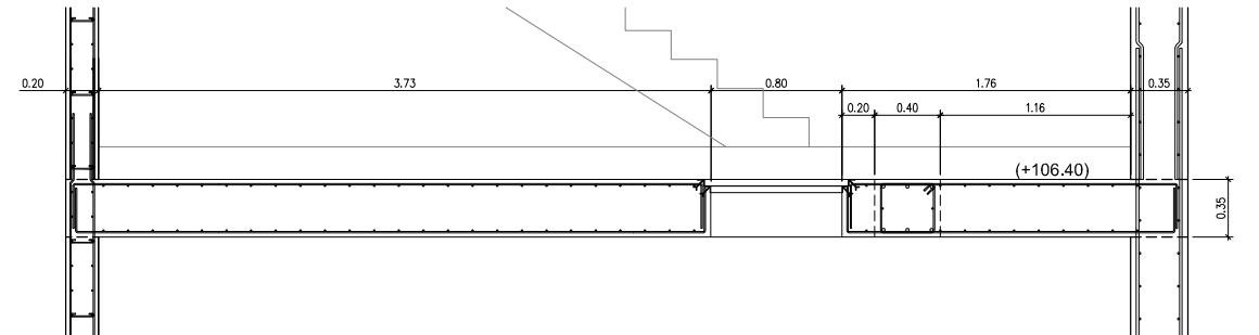
ESCALERA E1. DETALLE B5 Escala A1:1/25 - A3:1/50
