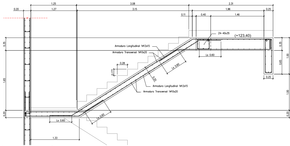
ESCALERA E1. DETALLE B1 Escala A1:1/25 - A3:1/50
