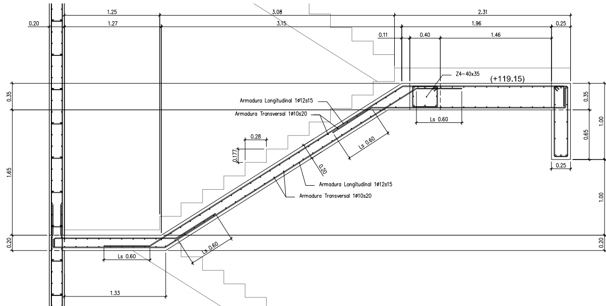
ESCALERA E1. DETALLE B2 Escala A1:1/25 - A3:1/50
