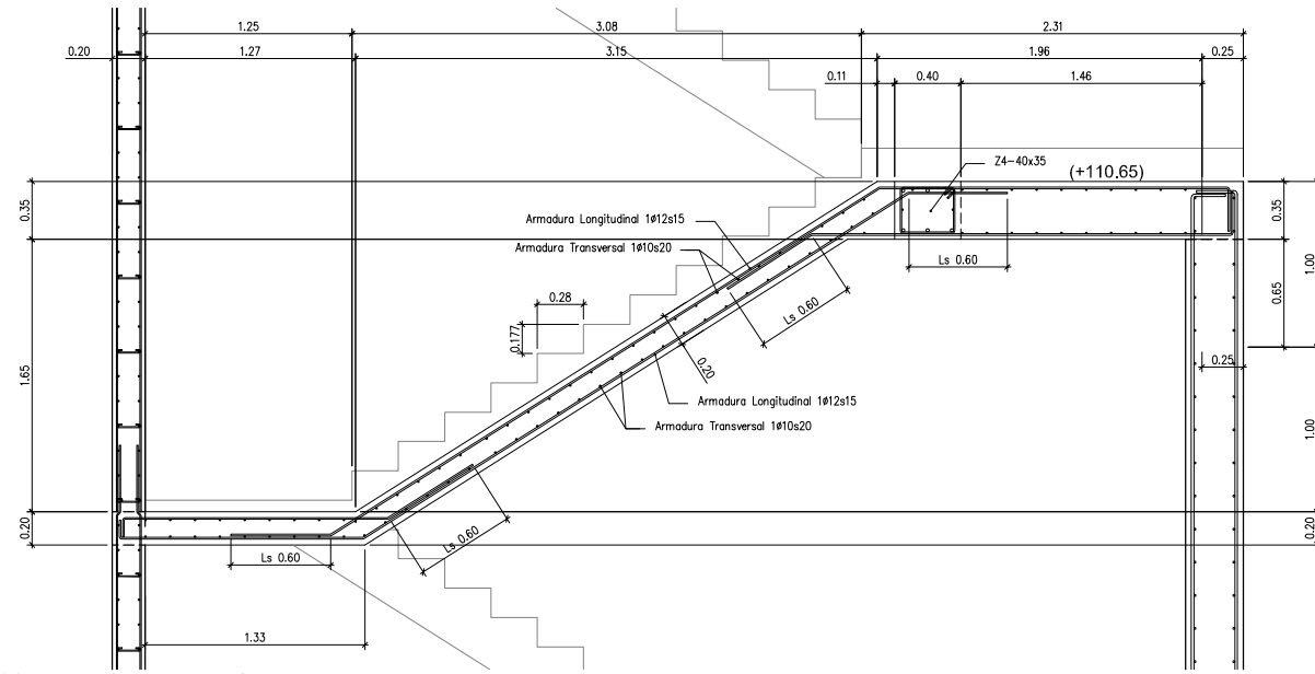
ESCALERA E1. DETALLE B4 Escala A1:1/25 - A3:1/50
