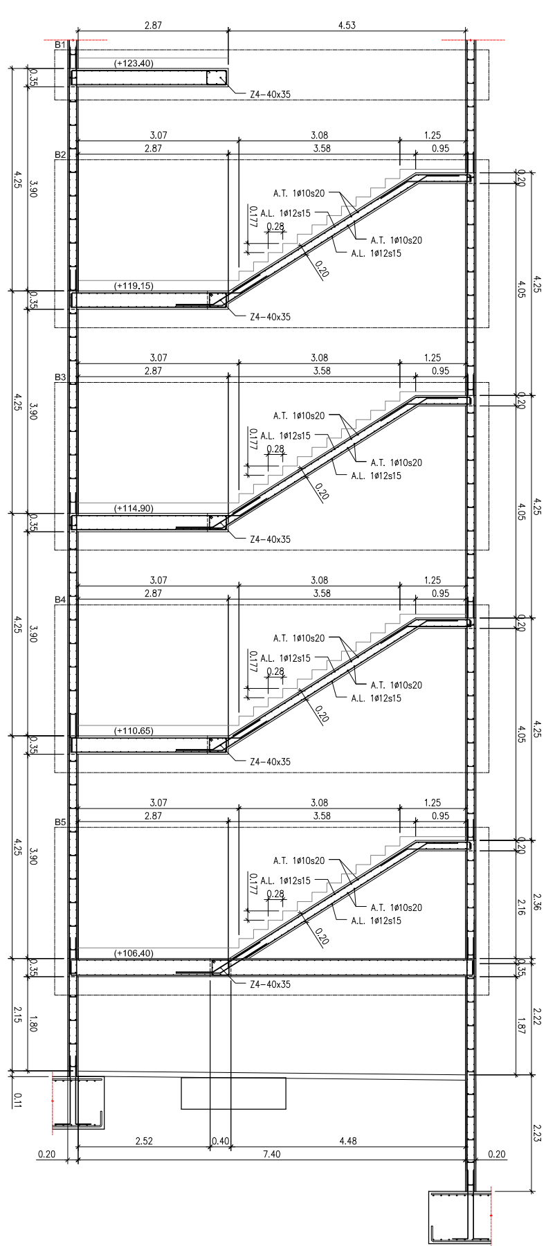
ESCALERA E2. SECCION A-A Escala A1:1/50 - A3:1/100
