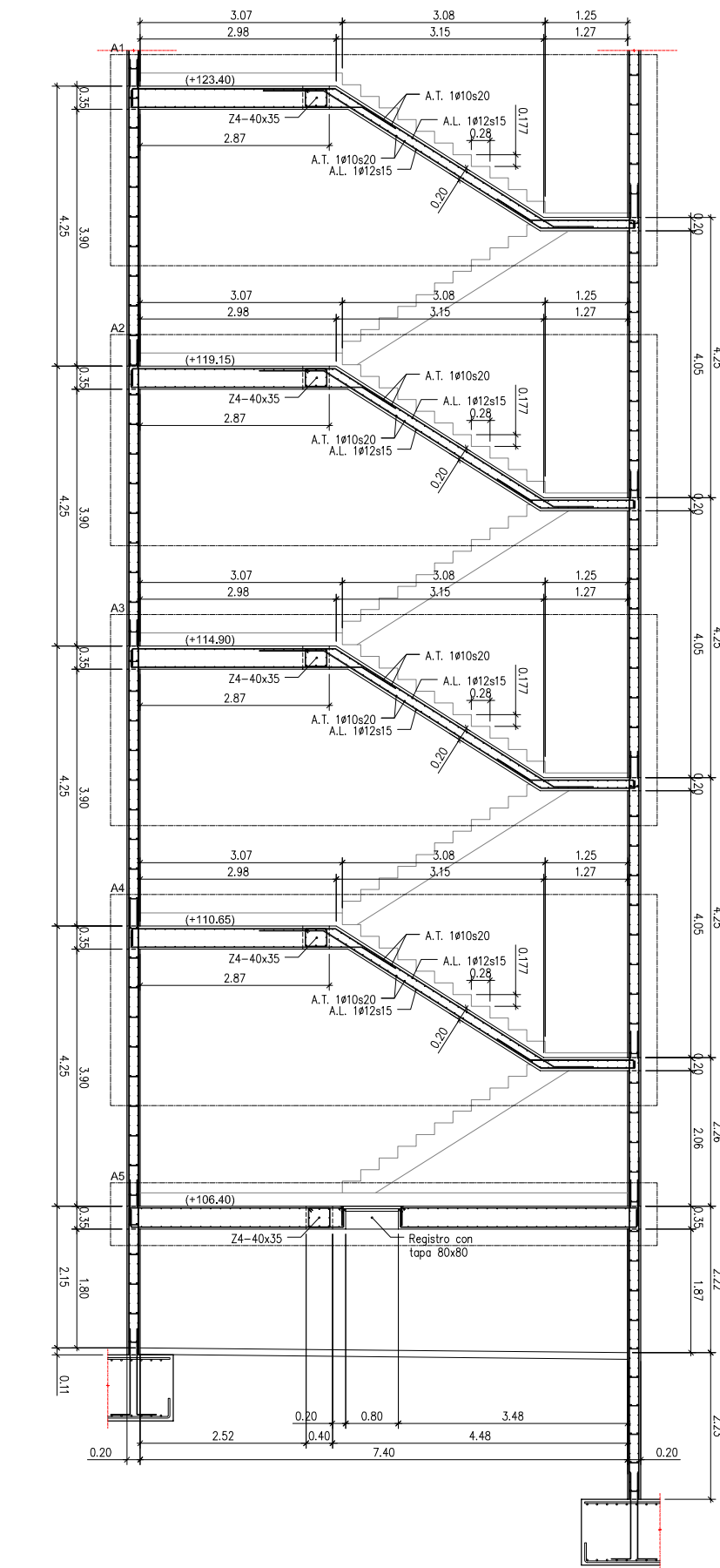
ESCALERA E2. SECCION B-B Escala A1:1/50 - A3:1/100
