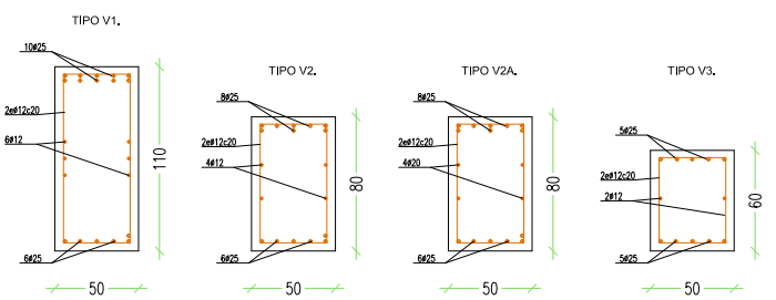
VIGAS 1:25
